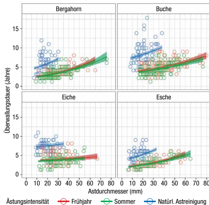
Abb. 6: Zusammenhang zwischen Überwallungsdauer und Astdurchmesser
